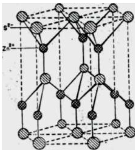
Fig. 1.2 Wurtzite ( \text{ZnS} ) Structure
